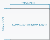
Cutout Dimensions
