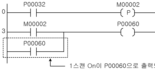
[ 래더 프로그램 ]
