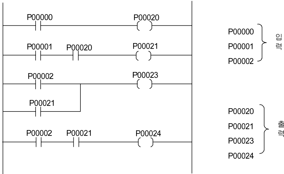
그림 2.1 입출력 회로 구성예
